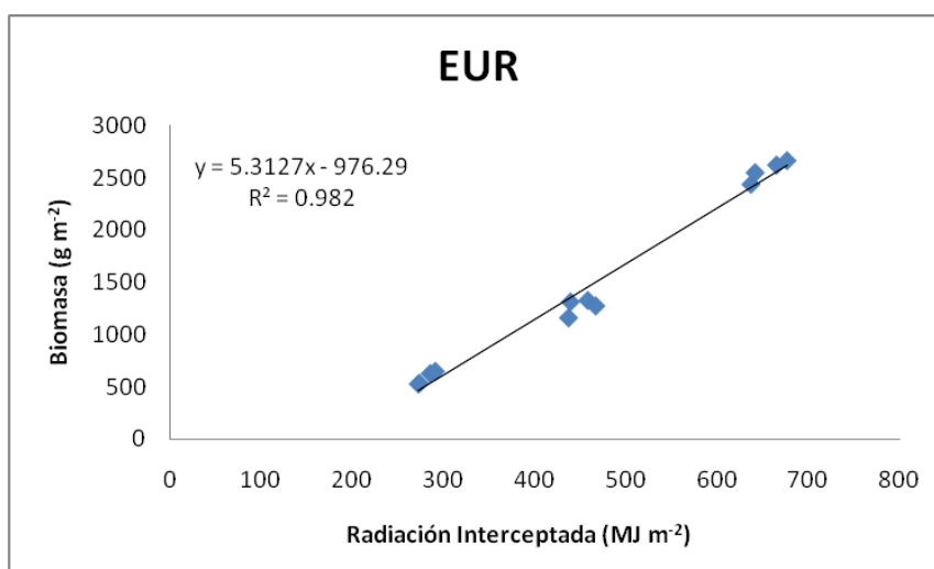
Figura 4. Eficiencia de uso de la radiación (EUR) correspondiente a los cuatro híbridos durante el ciclo productivo.
