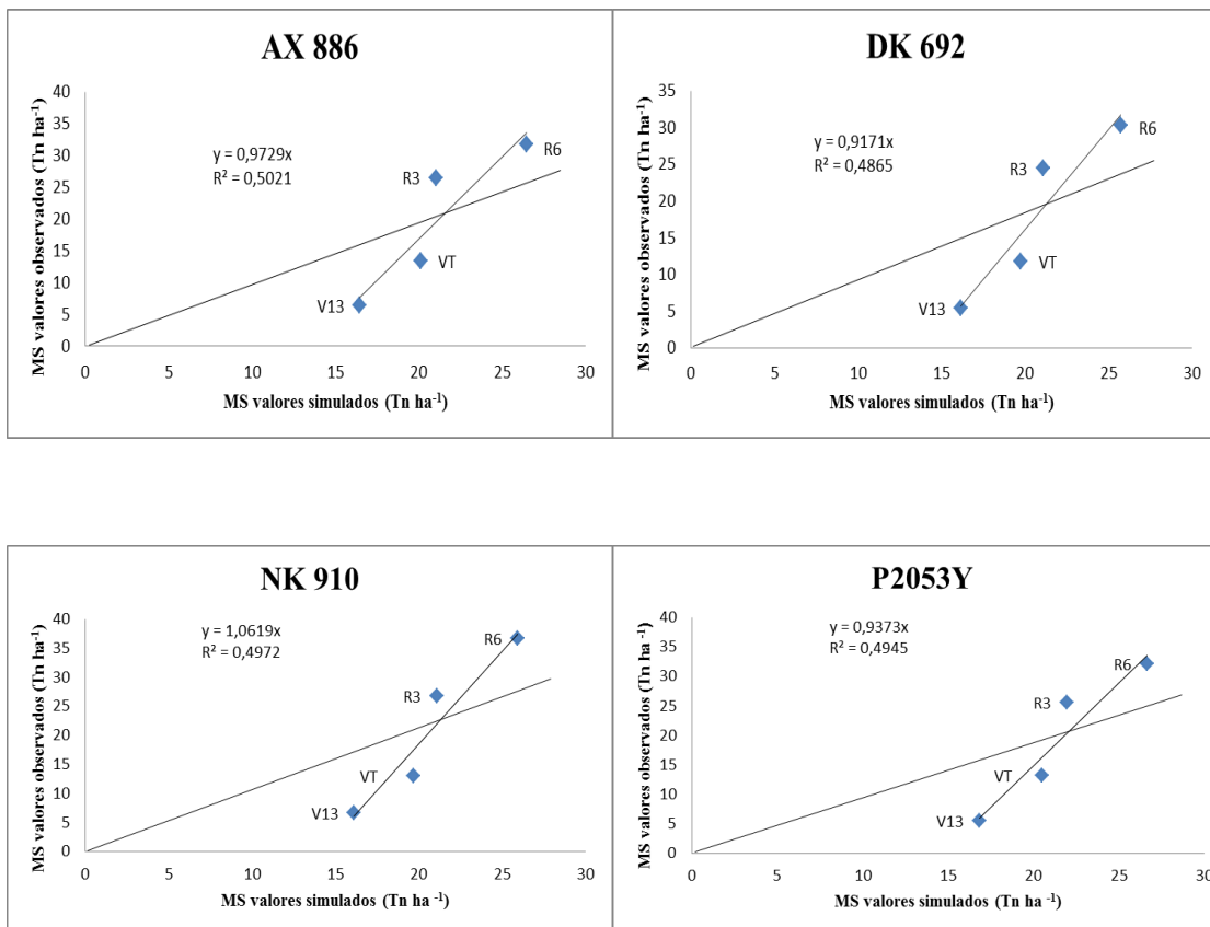
Figura 5. Valores simulados y observados de producción de materia seca total (Tn MS ha -1 ) correspondiente a cada híbrido a lo largo del ciclo productivo.
