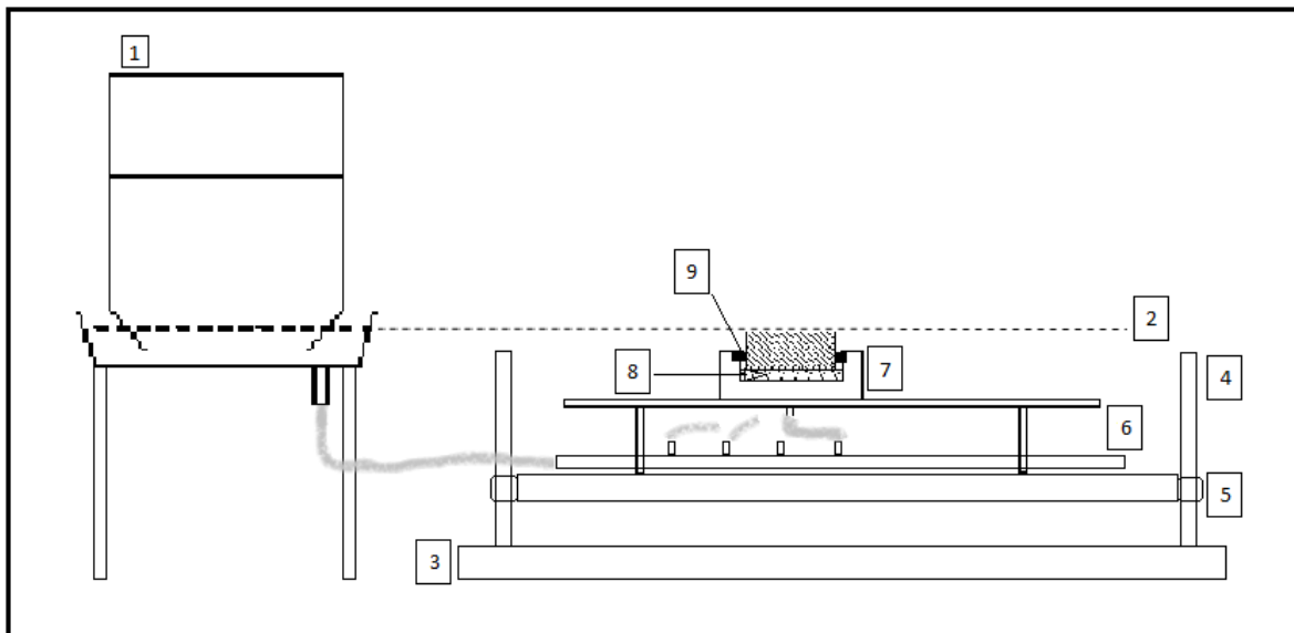
Figura 2.2 Esquema del dispositivo de vasos comunicantes para saturar las muestras y la mesa de tensión diseñada para determinar cualquier porosidad mayor a 75\mu .
